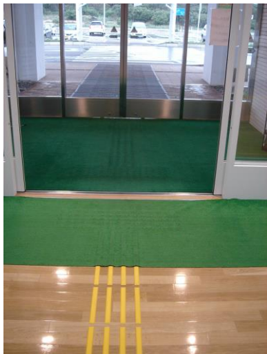
21-5 施設の入口の点字ブロック上に、泥除けのためにマットを敷いているケースがしばしばある。しかし、マットによってブロックの突起が確認しづらくなるため、ブロック上にマットを敷いてはいけない。（奥尻空港）
